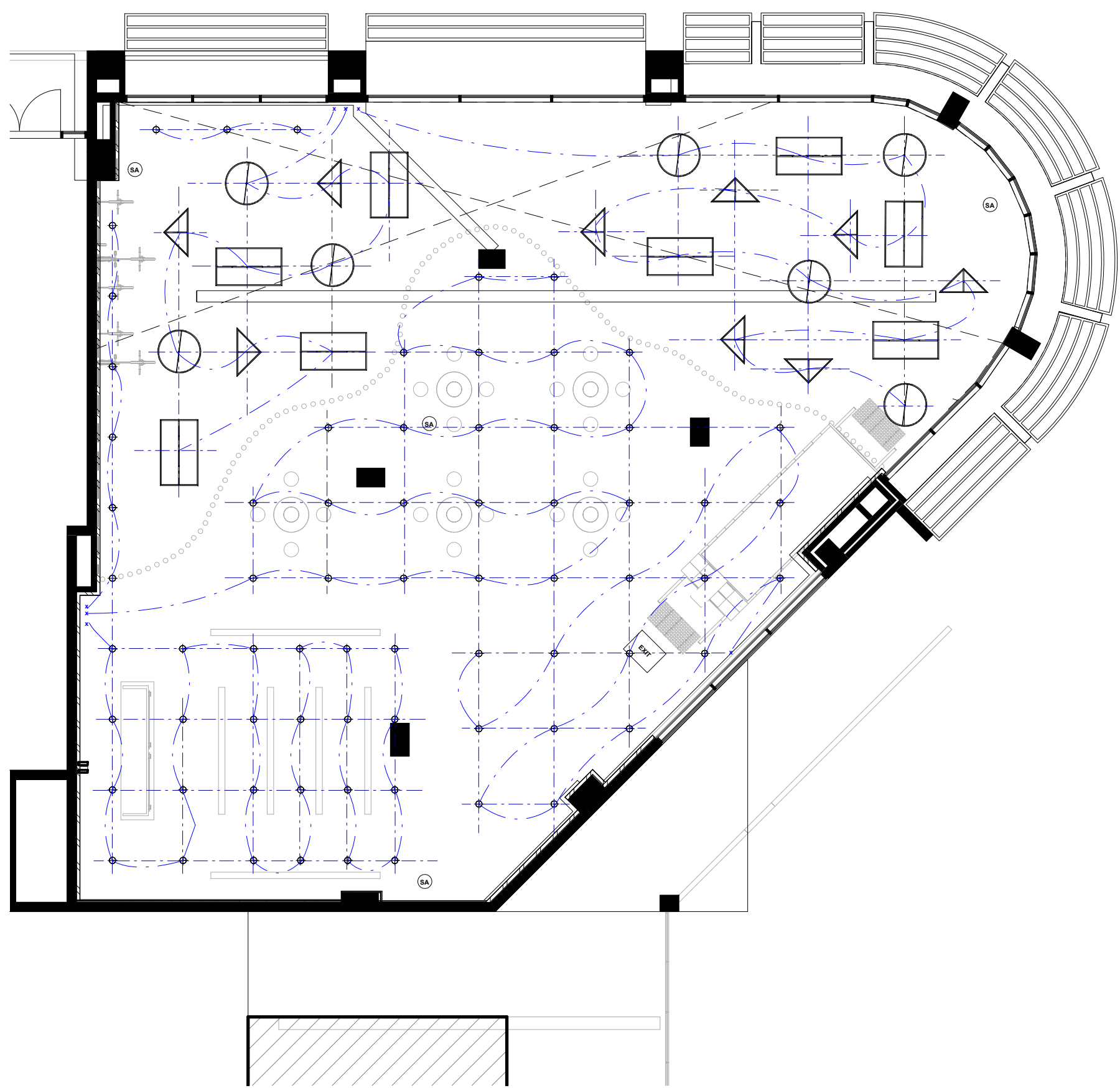
1 Level 2 RCP 1 : 100
