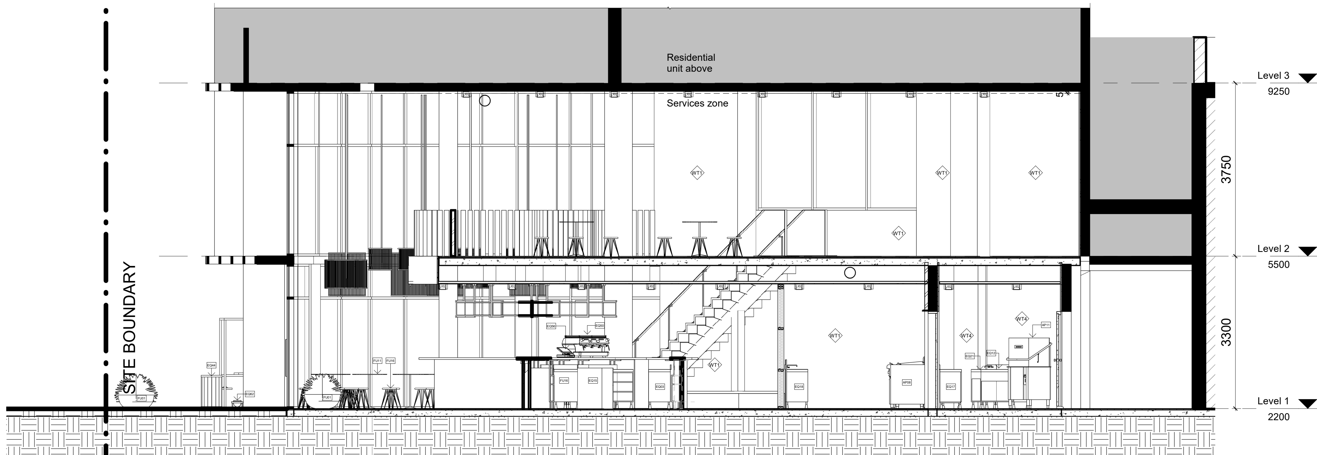
1 Section 1 1 : 50
