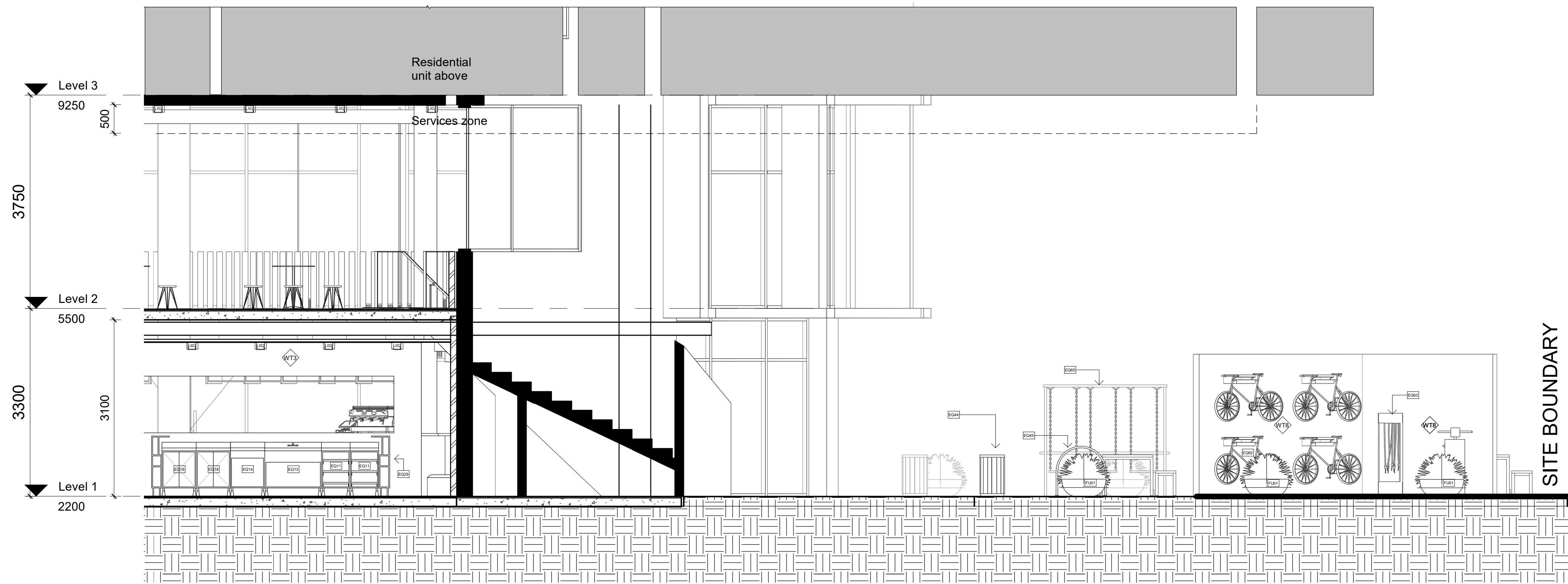
1 Section 2 1 : 50
