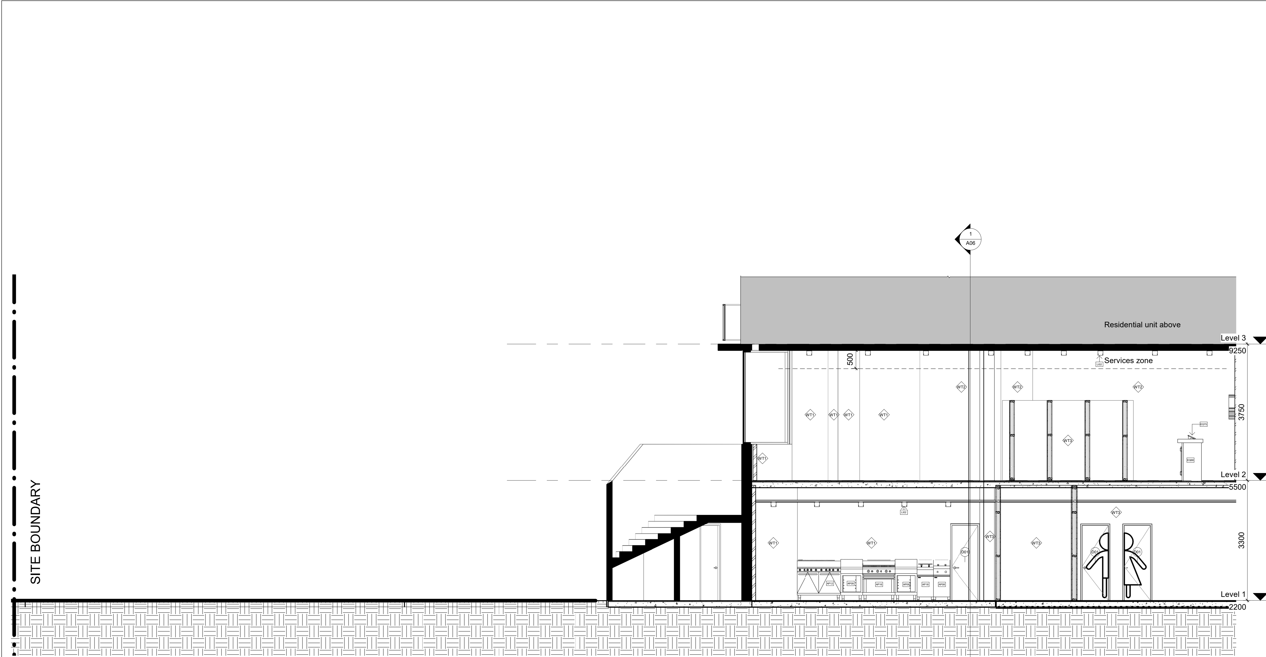
1 Section 3 1 : 50
