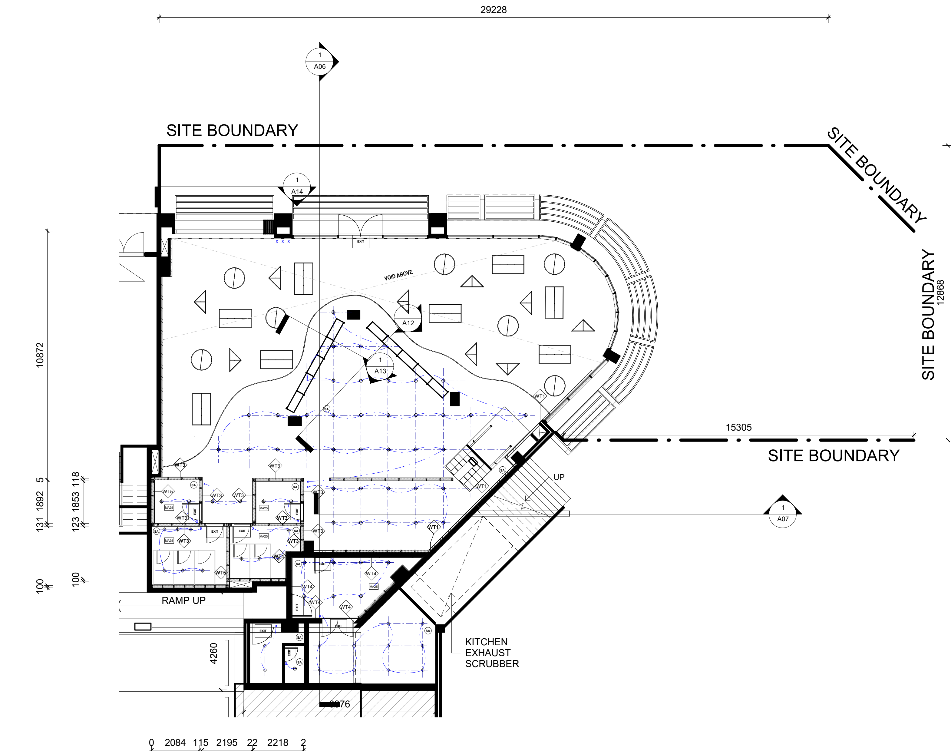
1 Level 1 RCP 1 : 100
