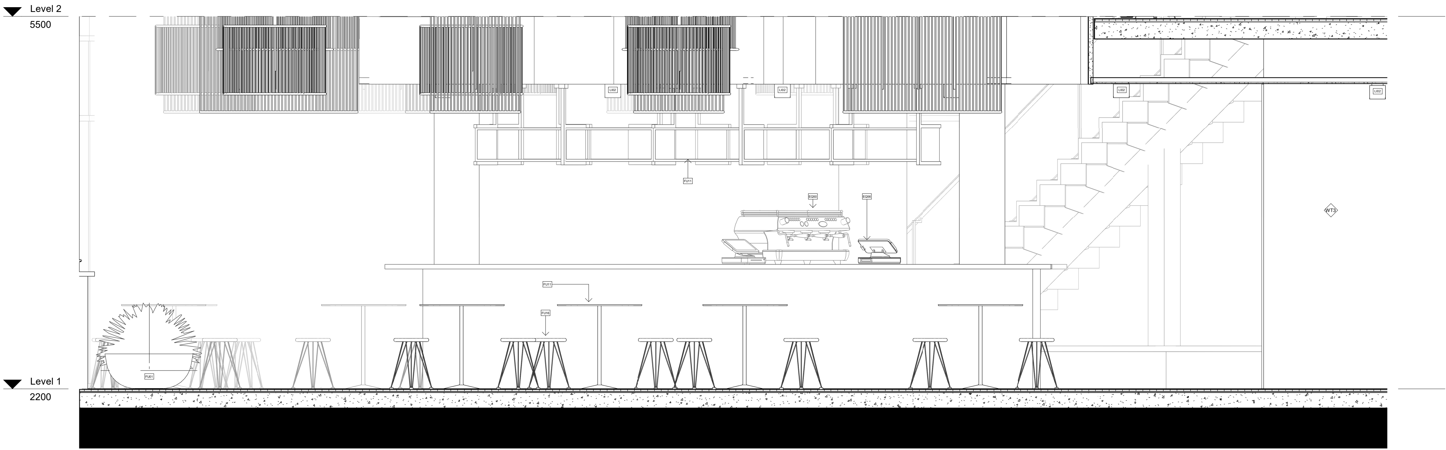
1 Bar Elevation 1 1 : 20
